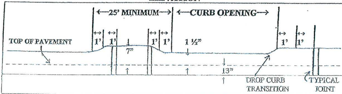
ELEVATION
